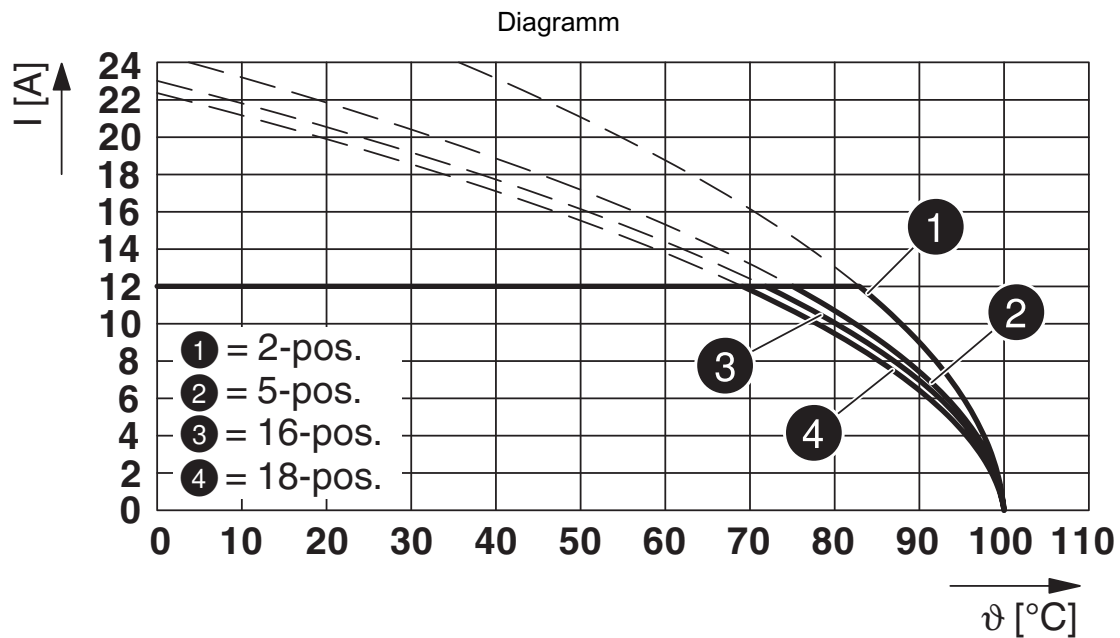
Typ: FKCVR(W/R) 2,5/...-ST mit SMSTBA 2,5/...-G
