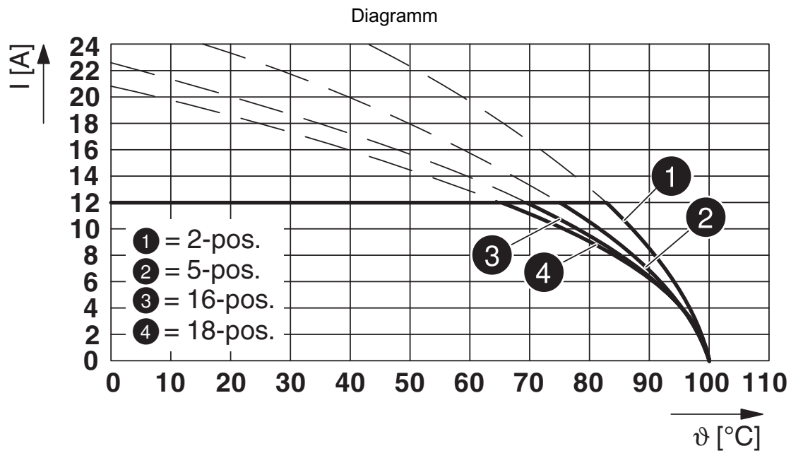
Typ: FKCVR(W/R) 2,5/...-ST mit MSTBW 2,5/...-G
