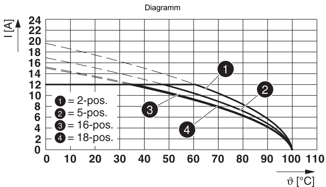
Typ: FKCVR(W/R) 2,5/...-ST mit MSTBVA 2,5/...-G
