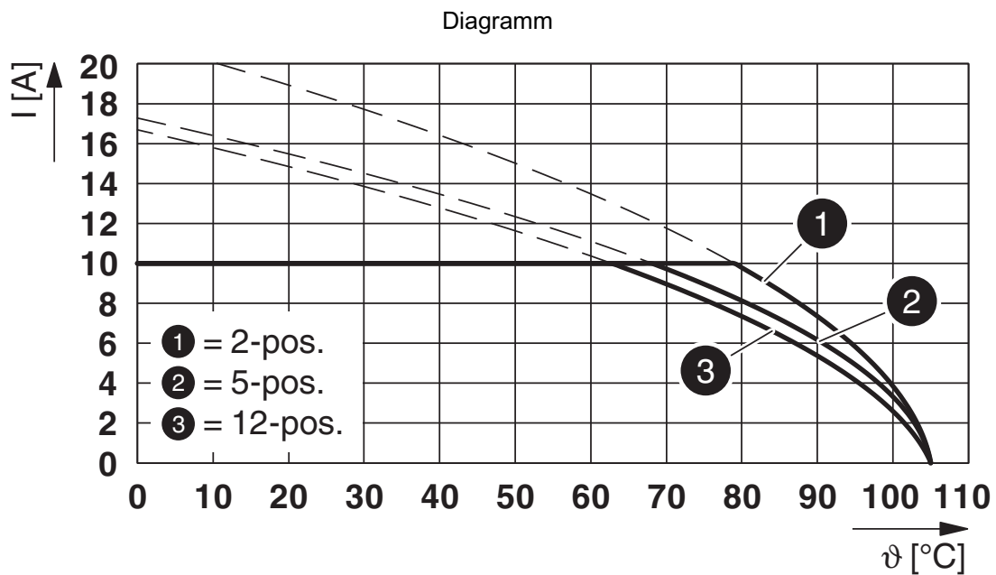
Typ: FKCVR 2,5/...-ST mit MDSTBVA 2,5/...-G
