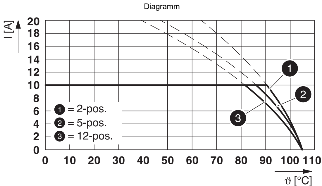
Typ: FKCVR 2,5/...-ST mit MDSTBA 2,5/...-G
