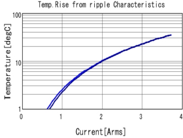
■ GRT155R61A475ME13 Temp. rise ■ 500kHz ■ 1MHz
