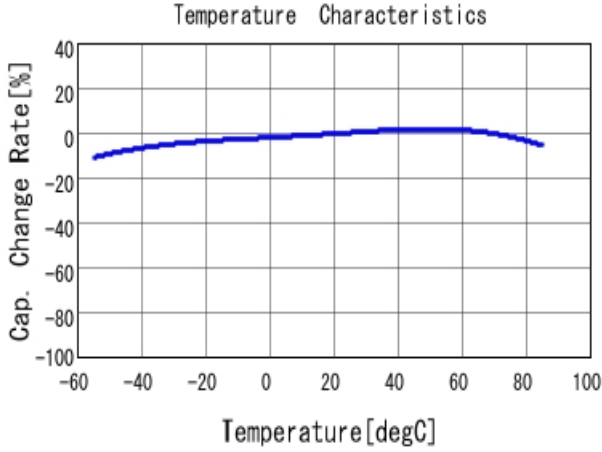
■ GRT155R61A475ME13 C-Temp. capchange, DCO. 0V, ACO. 1Vrm
