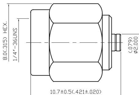
Dimensions : Millimetres (Inches)
