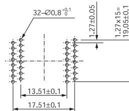
SOP IC51-0322-667-2 (32 Pins)
