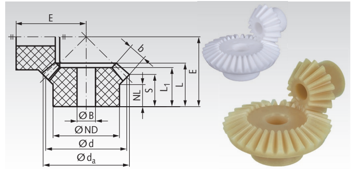
Zeichnung zeigt Übersetzung 1:1, Foto zeigt Übersetzung 2:1
