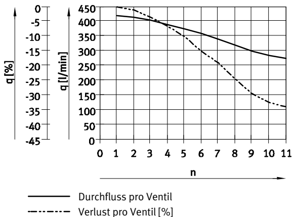
Durchfluss q pro Ventil bei mehreren (n) zeitgleich geschalteten Ventilen (Toleranz ± 20%)
