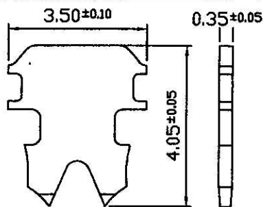
"1": 2 PRONGS FOR STRANDED WIRE 多芯線用二叉型金片
