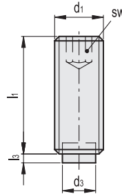
GN 913.5-KU
