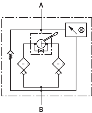
Filtre double avec by-pass et indicateur mécanique
