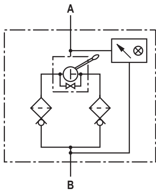
Filtre double sans by-pass et avec indicateur mécanique
