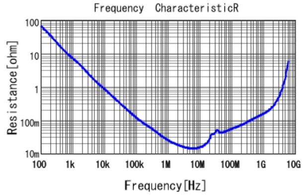
■ GCJ188R91E394KA01 R DC0V, 25degC
