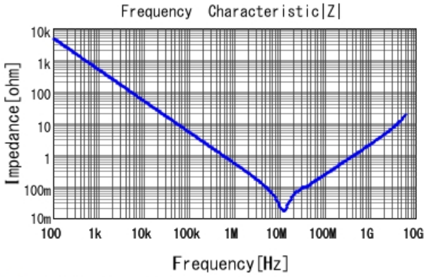
■ GCJ188R91E394KA01 |Z| DC0V, 25degC
