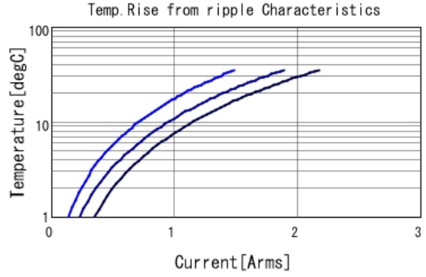
GCJ188R91E394KA01 Temp. rise ■ 300kHz ■ 600kHz ■ 1MHz
