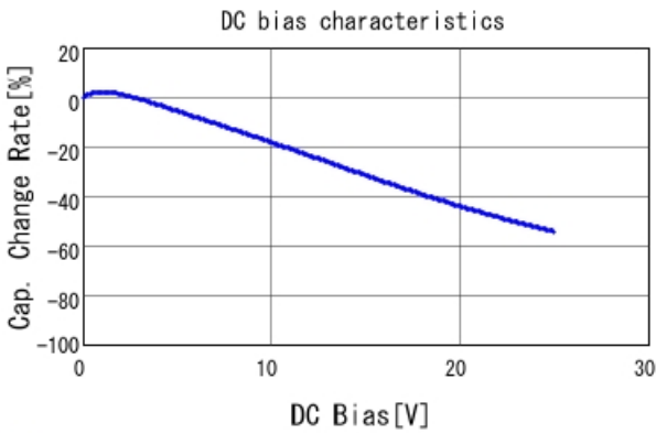
■ GCJ188R91E394KA01 C-DC bias capchange, 25.0degC, AC1.
