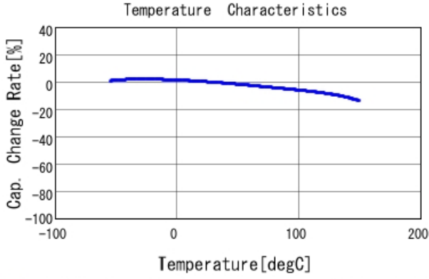
■ GCJ188R91E394KA01 C-Temp. capchange, DCO. 0V, AC1. 0Vrm
