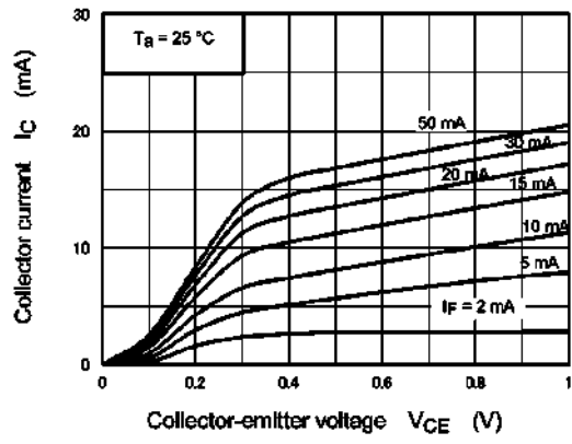
Fig. 11.8 I_C - V_{CE}
