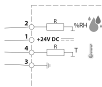
analog 4-20 mA
