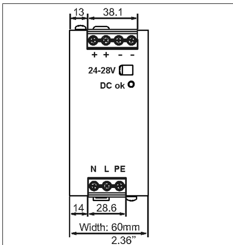
Bild 20-1 Vorderansicht
