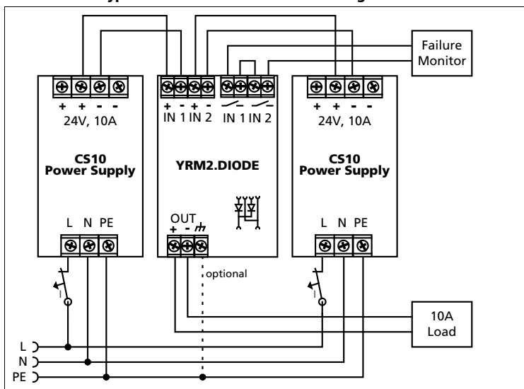
Bild 21-1 Typische 1+1 redundante Verschaltung für 10A Laststrom
