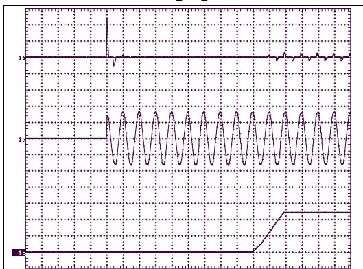
Bild 5-1 Typisches Einschaltstromverhalten Eingang
