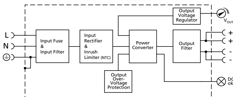
Bild 10-1 Funktionsschaltbild
