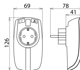
Maßbild DPRO 230
