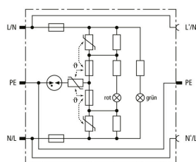
Prinzipschaltbild DPRO 230
