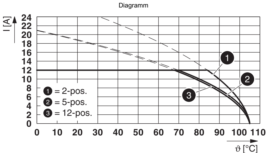
Typ: FKCS 2,5/...-STF-5,08 mit CC 2,5/...-GF-5,08 P...THR
