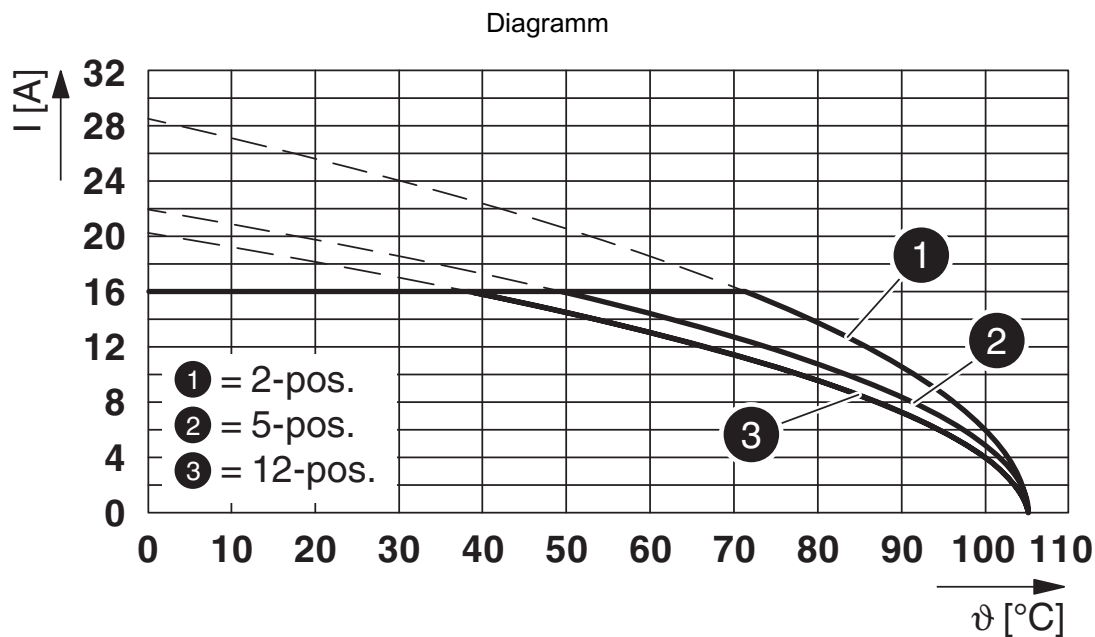
Typ: FK 2,5 HC/...-STF-5,08 mit CC 2,5/...-GF-5,08 P26THR
