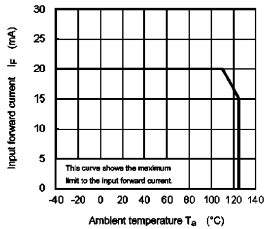
Fig. 12.2.2 I_F - T_a
