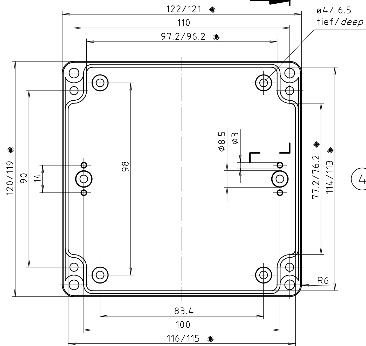
Unterteil / base
