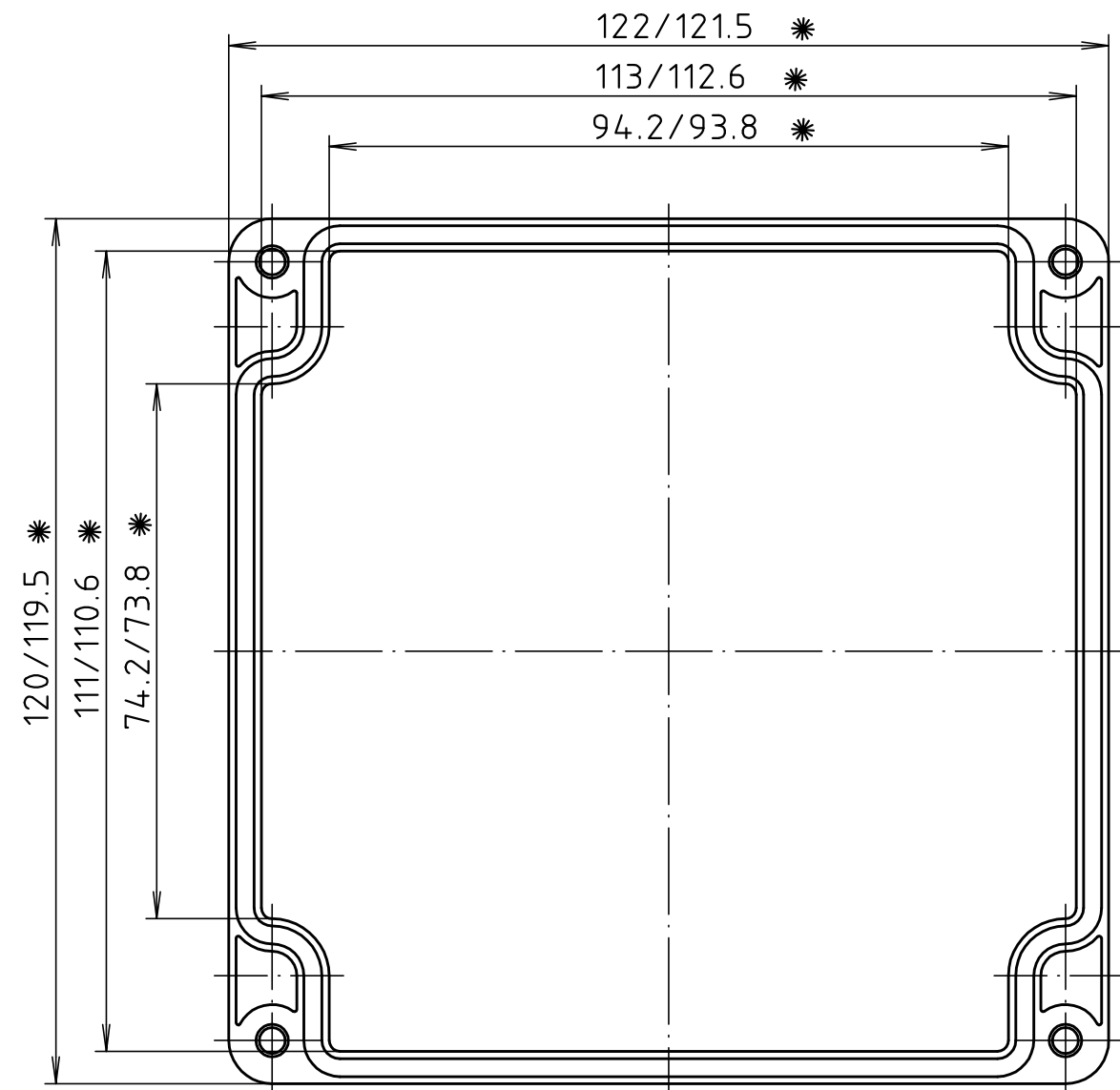
Deckel / lid
