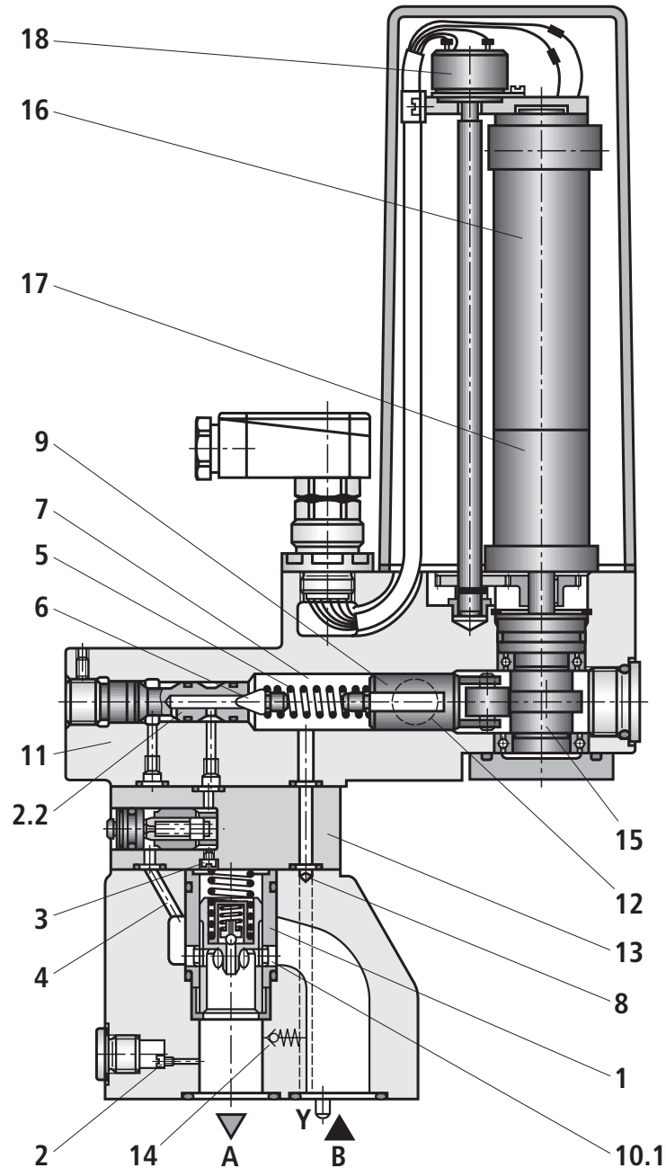
Type DRG 20-1X/..Y
