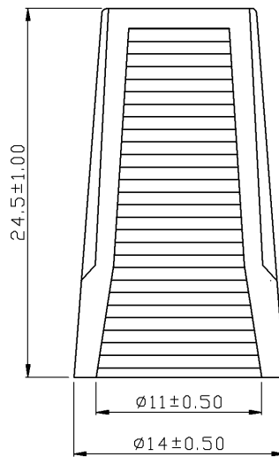
Dimensions : Millimetres
