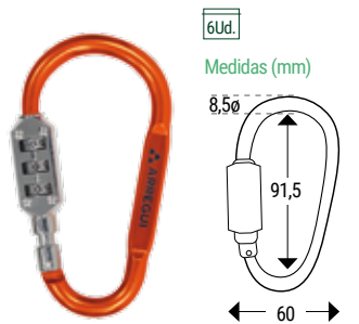
Mosquetón A-1313130
