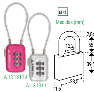
Arco flexible A-1313110 / A-1313111
