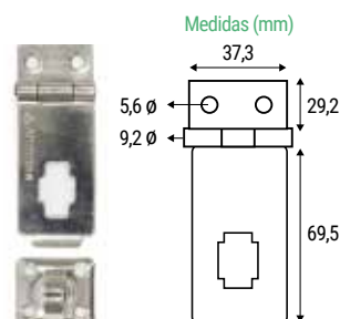
Mini Loop A-1313170
