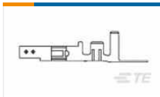
TE Teilnr.:794956-3 VAL-U-LOK SKT PHBZ SN 22-18AWG
