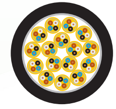
Schnittzeichnung
