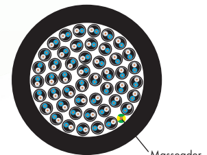
Schnittzeichnung
