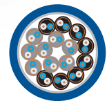
Schnittzeichnung
