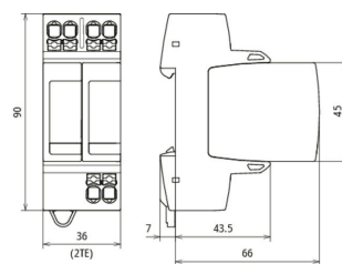
Maßbild DG MP TN 275
