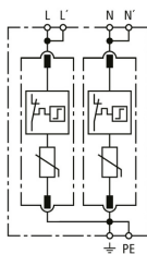
Prinzipialschaltbild DG MP TN 275
