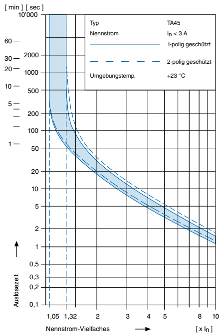
Auslösekennlinien I_n < 3 A
