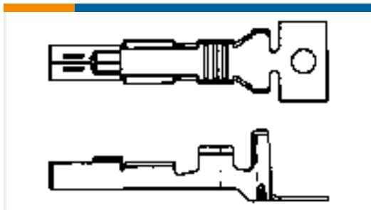
TE Teilenummer1123907-1 1.5 MINI CT LATTICE POWER REC
