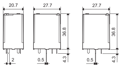
Typ 56.42/42-0300
