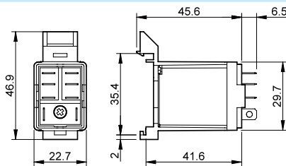
056.27 mit Relais
