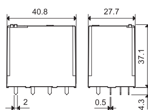
Typ 56.44
