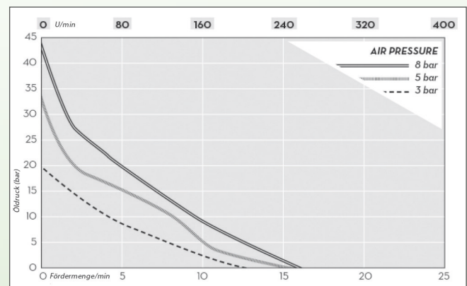
P 5.5 ST – P 5.5 940 Hohe Viscosität
