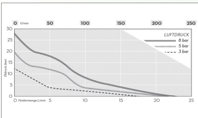
P 3.5 ST – P 5.5 940 Mittlere Viscosität
