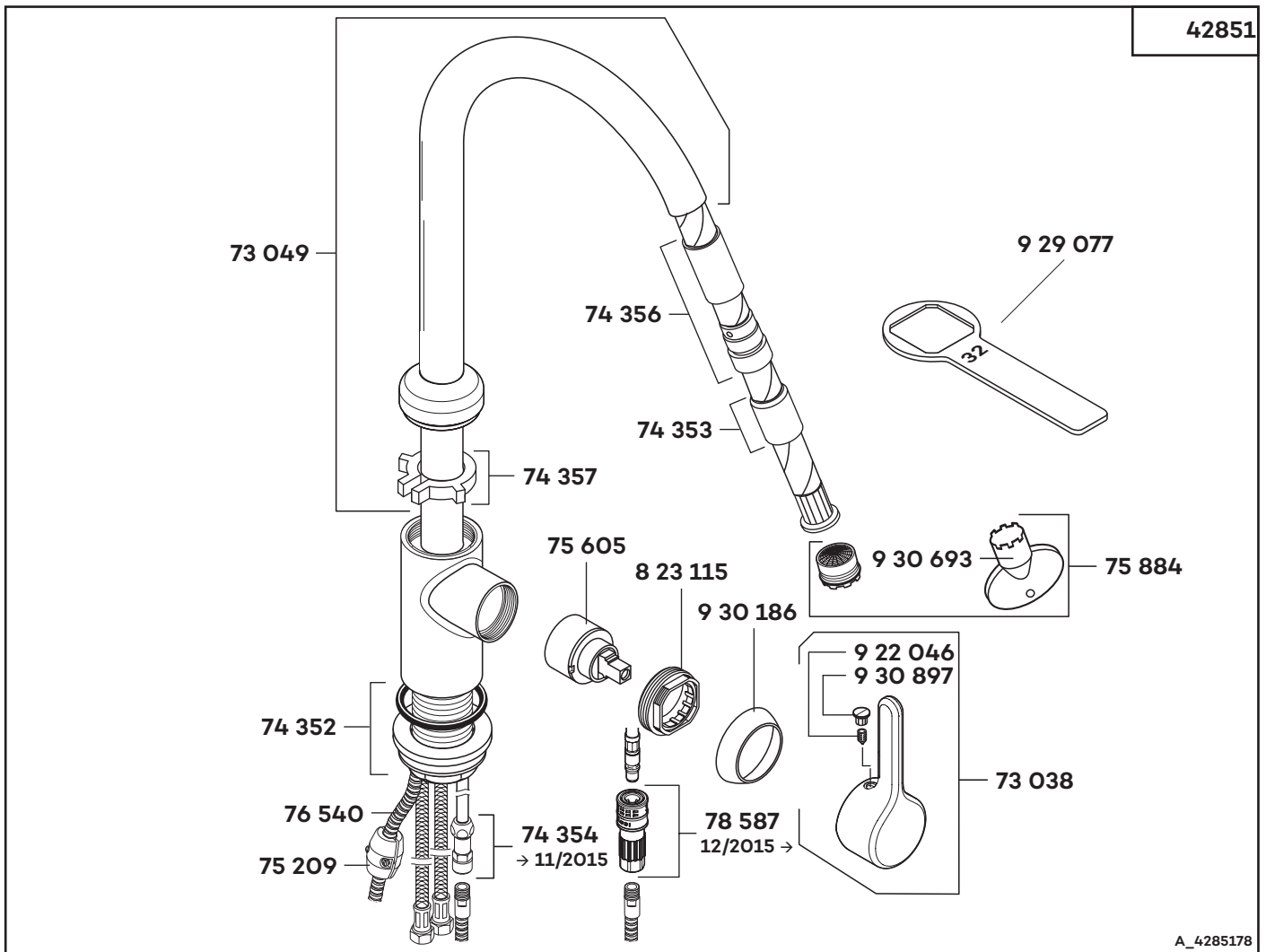
42851 Spültisch-Einhandmischer DN 15 single lever sink mixer DN 15 ééngreeps gootsteenmengkraan 1/2"
