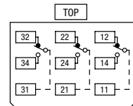
3PDT Contacts
