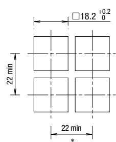
Square (LB7S/LB7MS)
