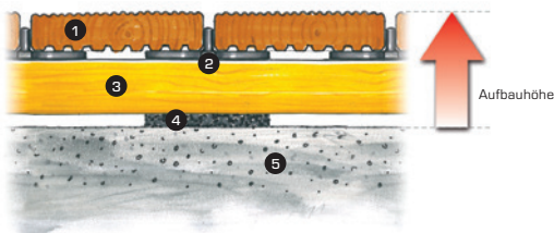
1 Holzbelag | 2 Abstandhalter | 3 Holz-Trägerbalken 4 Unterlage Pad | 5 Betonsockel/Streifenfundament
