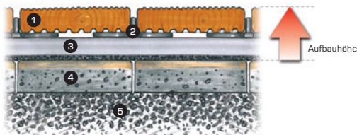
1 Holzbelag | 2 Abstandhalter | 3 TerraStep Schiene 4 Pflastersteine, alter Terrassenbelag | 5 Kies
