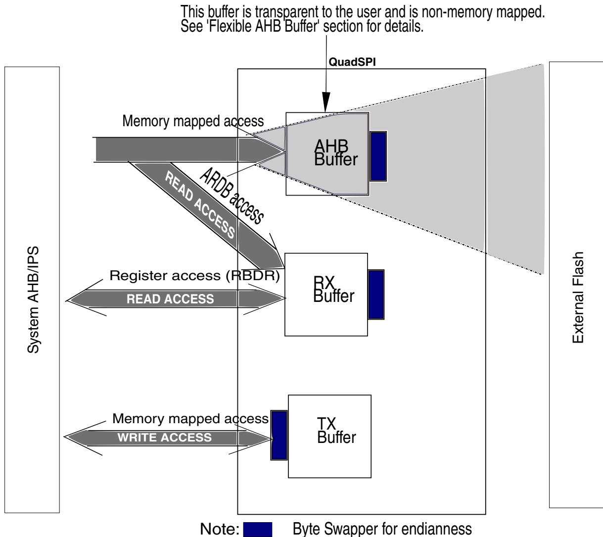
Figure 36-7. QuadSPI memory map
