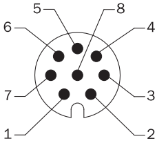
Ansicht Gerüstestecker M12 am Encoder
