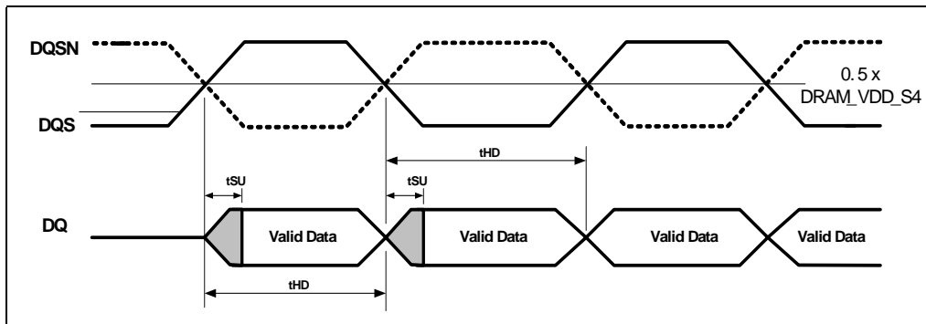
Figure 21. DDR3L DQ Setup/Hold Relationship to/from DQSP/DQSN (Read Operation)
