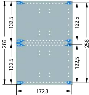
Tiefe 176 mm
