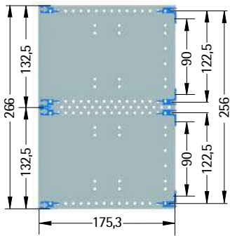
Tiefe 176 mm
