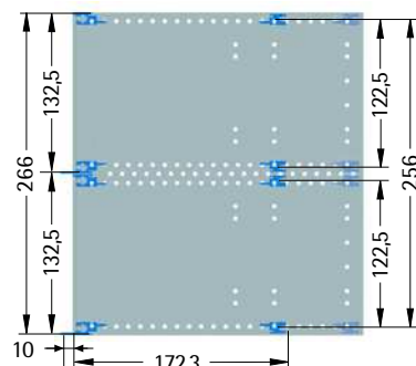
Tiefe 236 mm
