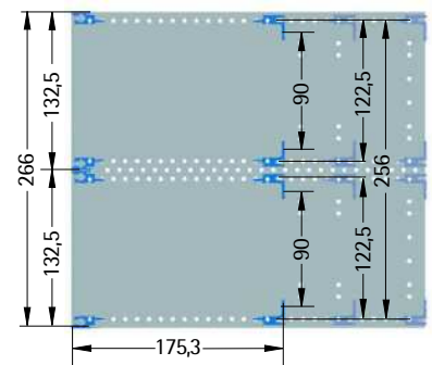
Tiefe 296 mm
