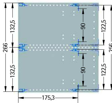
Tiefe 236 mm
