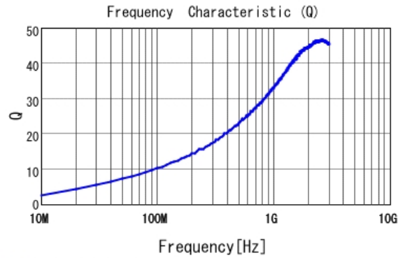
■ LQG15HS2N2S02 Q
