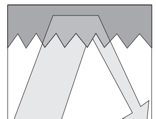
La placa de pirámides de espuma que absorbe el sonido
