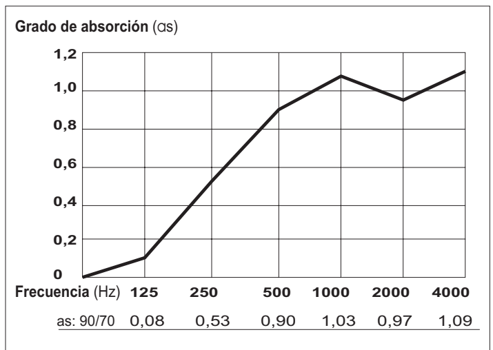
La placa de pirámides de espuma que absorbe el sonido
