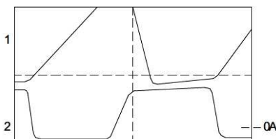
Dynamische Lastreaktion ohne Stromsenke: negativer Laststrom durch Rücker speisung entsteht
