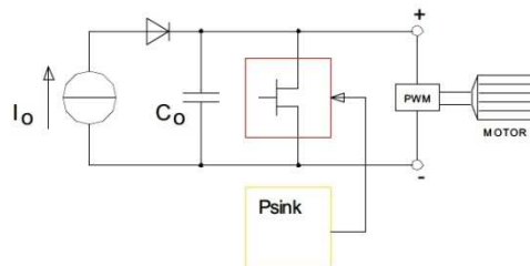
Mit Stromsenke (Psink): Bremsenergie wird absorbiert
