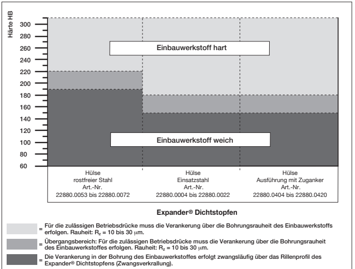
Abb. 1 Auswahldiagramm
