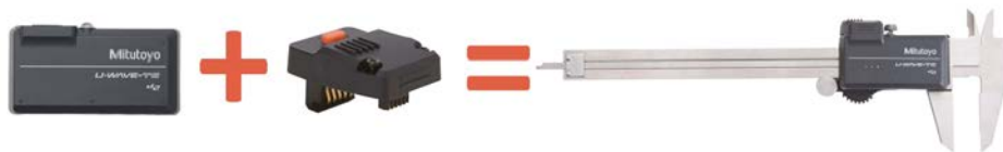
Adó és csatlakozó egység (lásd következő oldal) tolómérőhöz (U-WAVE-TC + 02AZF300)
