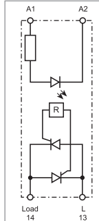
Prinzip-Schaltbild
