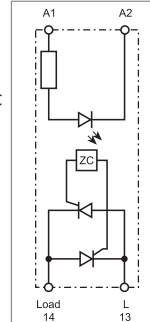
Prinzip-Schaltbild
