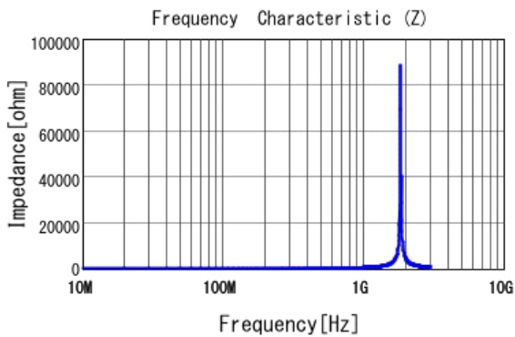
■ LQW2BAS68NG00 |Z|
