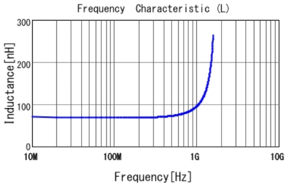
■ LQW2BAS68NG00 L
