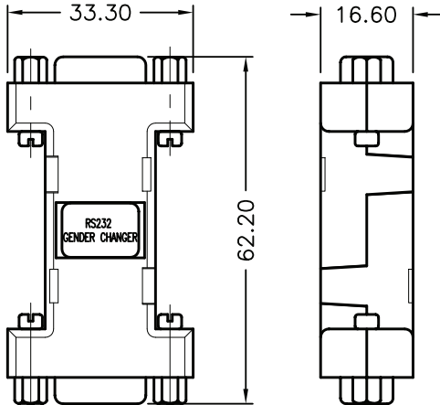
DB-9(F)
