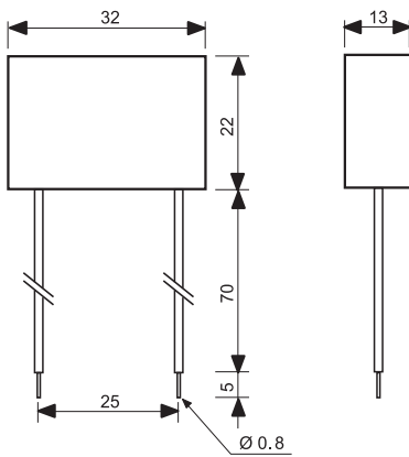
Tipo 026.00 Versione ermetica con reofori isolati e flessibili da 7.5 cm.
