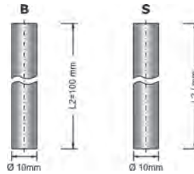
Halsrohr
