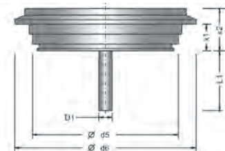
Typ R / P - Varivent®
