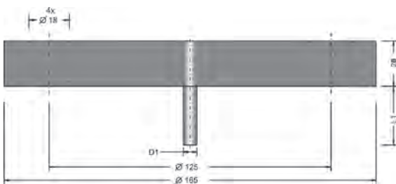
Fühler
