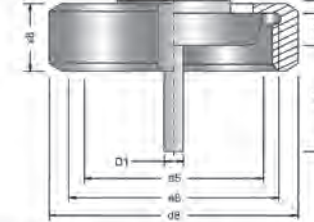
Typ M / N / O - DIN 11851
