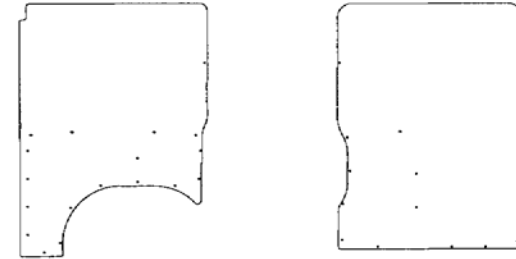
Seitenwand (links)
