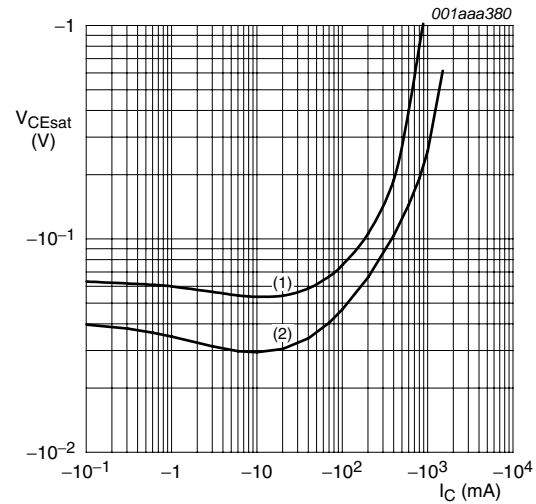
T_{amb} = 25^\circ C (1) I_C/I_B = 50 (2) I_C/I_B = 20
