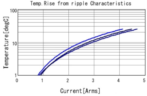
KRM55WR72A226MH01 Temp. rise ■ 50kHz ■ 100kHz ■ 300kHz
