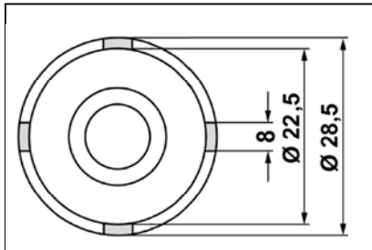
Abmessungen KL-0369-601
