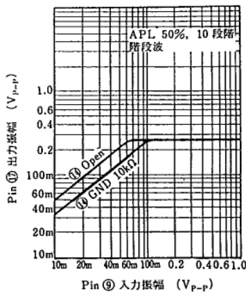
AGC アンプ入出力特性
