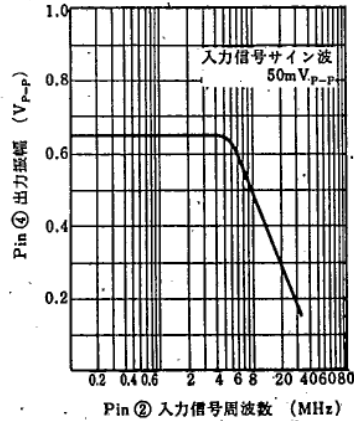
クロマアンプ周波数特性
