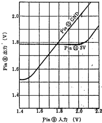
Y_L 入出力特性
