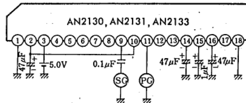
Test Circuit 7 ( v_{O(LAG1)} , v_{O(LAG2)} , v_{O(LAG3)} , v_{O(ABO-1)} , v_{O(ABO-2)} )
