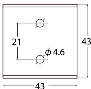
Lame de rechange BKT-300P, vue détaillée
