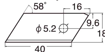
Lame de rechange BZL11P, vue détaillée
