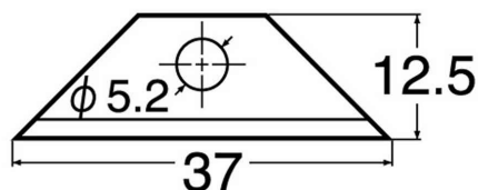
Lame de rechange BR-400P, vue détaillée
